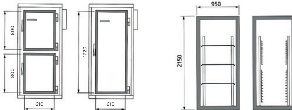
Dimensiones puertas
